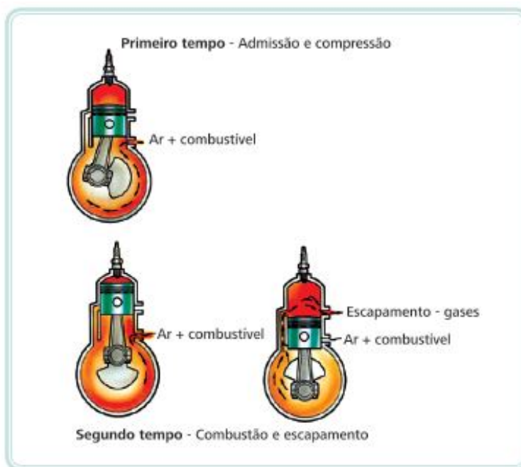
Figura 1: Funcionamento motor 2 tempos – ciclo Otto. Fonte: MAHLE, 2016
