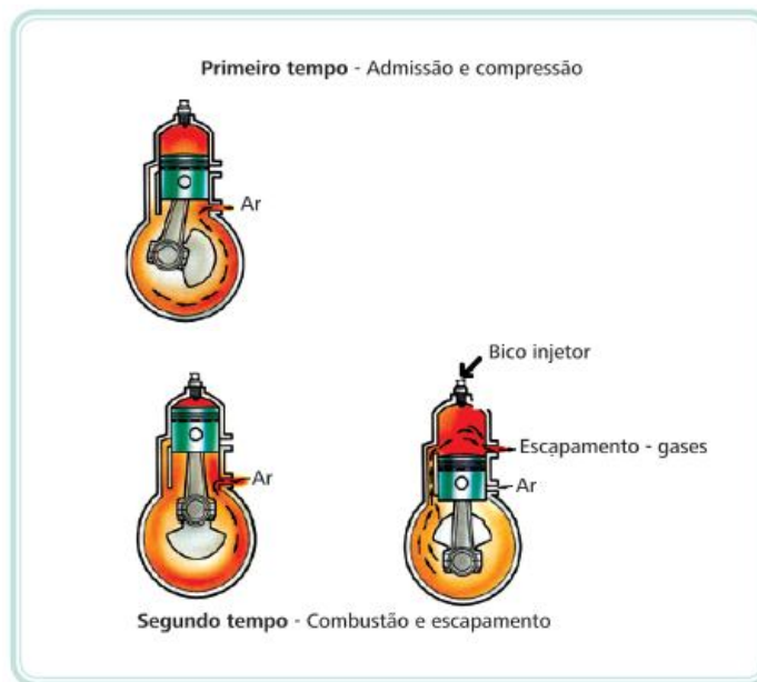
Figura 2: Funcionamento do motor 2 tempos – ciclo Diesel. Fonte: MAHLE, 2016
